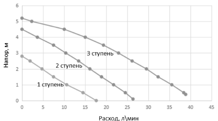
Рис. 13. Напорная характеристика насоса.
