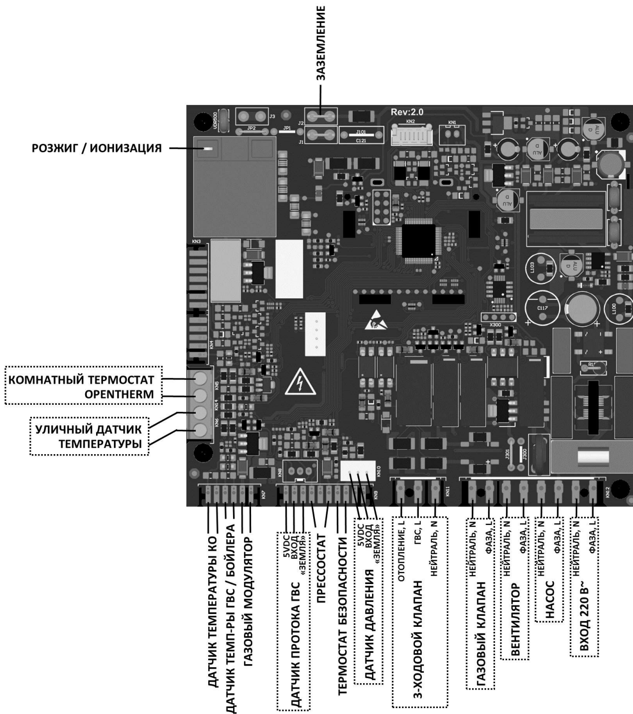
Рис. 14. Электрическая схема
